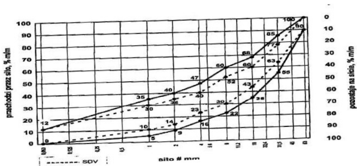
rys. 1 Uziarnienie mieszanki niezwiązanej 0/63 do podbudowy
