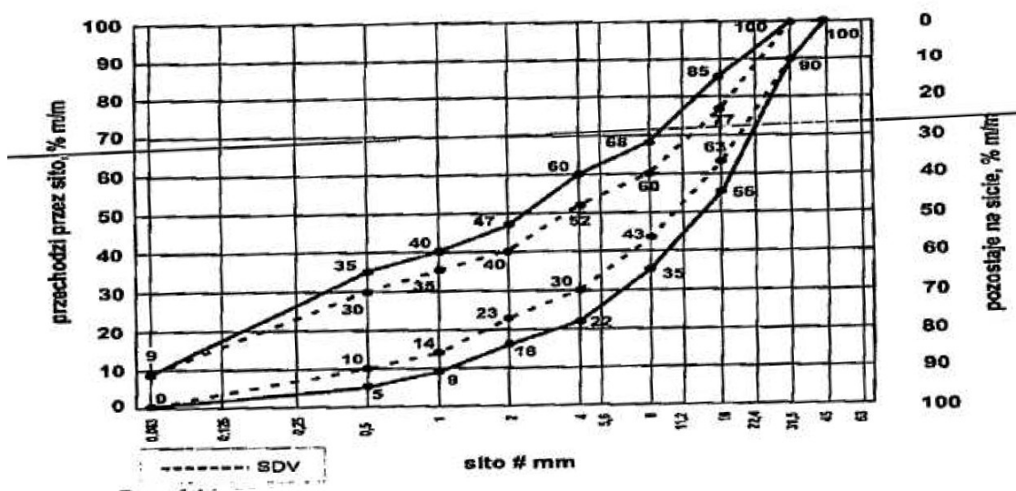
rys. 3 Uziarnienie mieszanki niezwiązanej 0/31,5 do podbudowy
